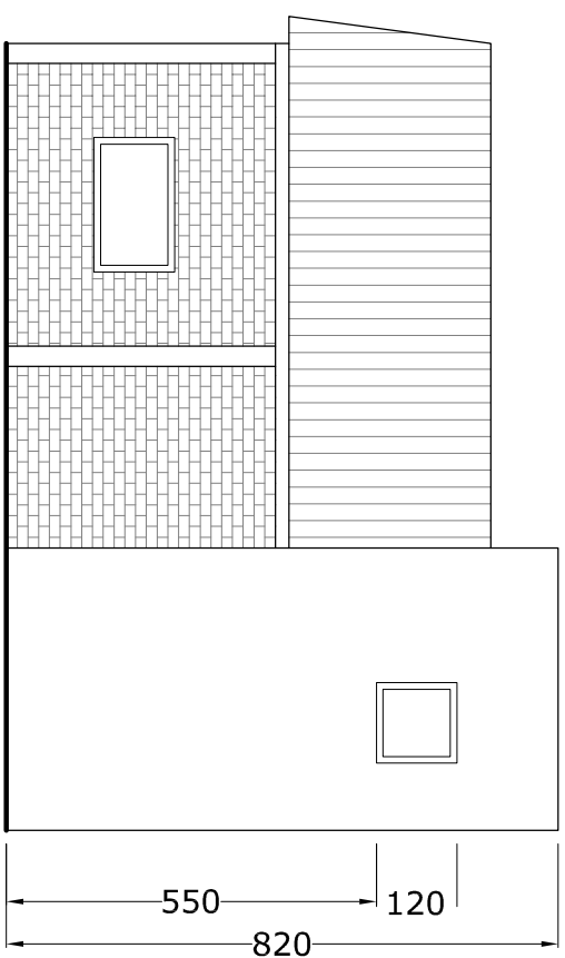
PROSPETTO EST
